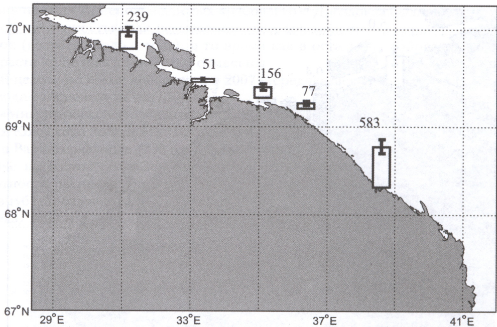
Рис. 6. Средняя плотность распределения неполовозрелых особей камчатского краба (экз/1000 м 2 ), исключая сеголеток, в прибрежной зоне Кольского п-ва в июне 2007 г.
