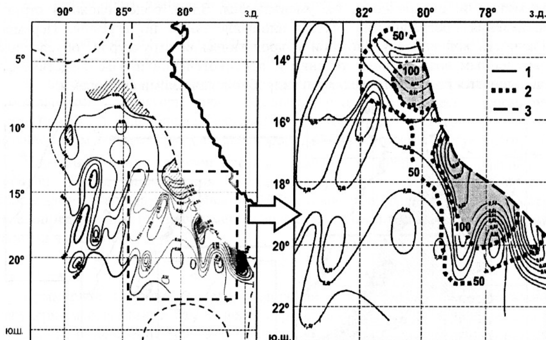
Рис. 1. Распределение величины e_{675} на глубине 20 м (слева) и участок сравнения с плотностью рыбных скоплений (справа): 1 – ослабление света; 2 – плотность рыбных скоплений (т/миля 2 ); 3 – граница НРЗ Перу.
