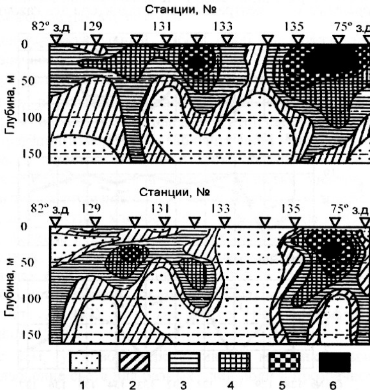
Рис. 4. Вертикальное распределение пигментного поглощения по данным ЛФП-2 (вверху, усл.ед.), а также золотистых и перидиниевых водорослей (внизу, мг/м 3 ): 1 – менее 1; 2 – 1-5; 3 – 5-10; 4 – 10-25; 5 – 25-150; 6 – > 150.
