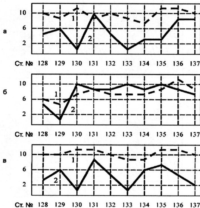
Рис. 5. Сравнительное распределение по станциям численности водорослей в слое 0-100 м (1; по вертикали в lg) и коэффициентов корреляции с k_f (2; по вертикали \times 0,1 ): а – золотистые и перидиниевые; б – перидиниевые; в – золотистые.
